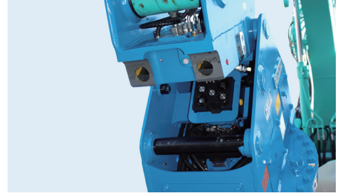
取付例
